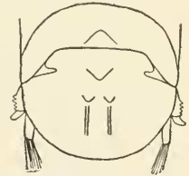
FIG. 21.—LIMNORIA JAPONICA. ABDOMEN. \times 15\frac{1}{2} .
